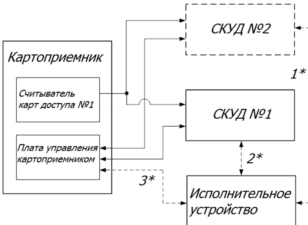
Рис. 11. Структурная схема №2
