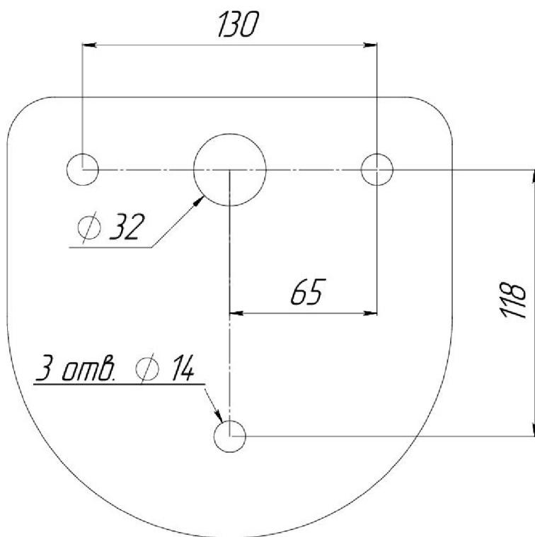
Рис. 3. Установочные размеры
