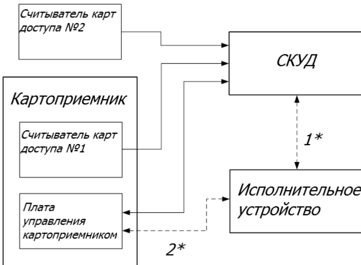
Рис. 10. Структурная схема №1
