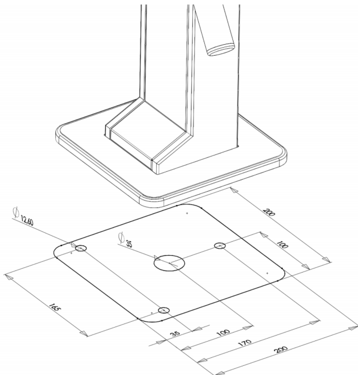
Рис. 17. Расположение монтажных отверстий и габариты турникета
