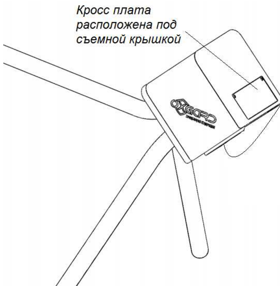
Рис. 10. Расположение кросс-платы на стойке турникета
